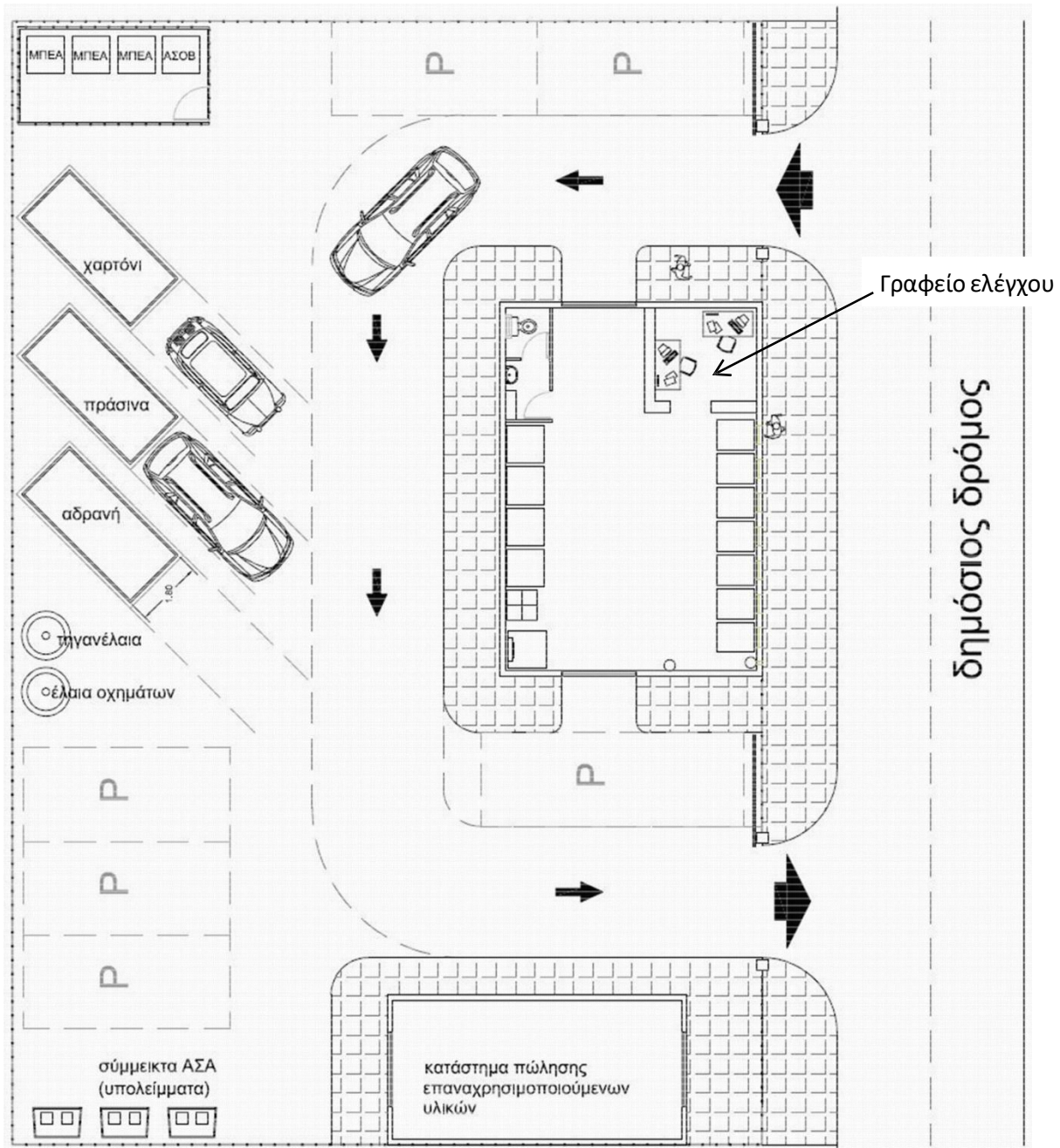
Σχέδιο 1: Ενδεικτική γενική διάταξη μικρής κλίμακας σταθερού ΠΣ σε χώρο έκτασης 600 τ.μ.
